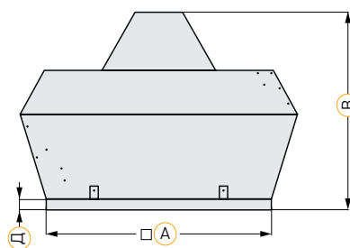
Типоразмеры 94-100
