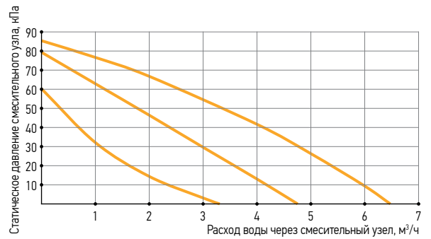
ONX 80-10,0
