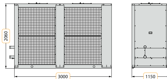
Типоразмеры 130-250
