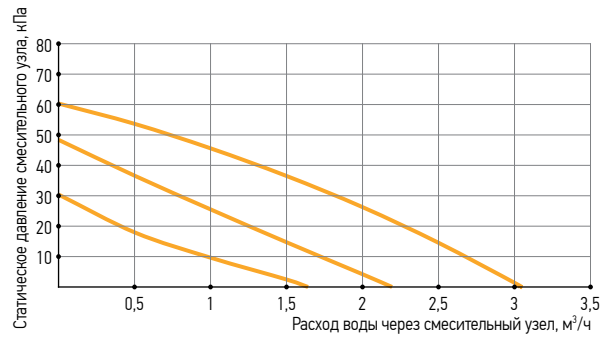
ONX 60-6,3
