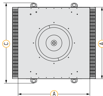
Вид снизу
