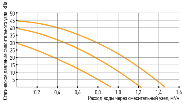
ONX 40-2,5
