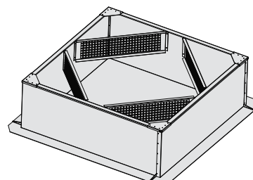
Общий вид типоразмеров 1120-1250
