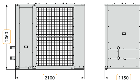
Типоразмеры 090-115
