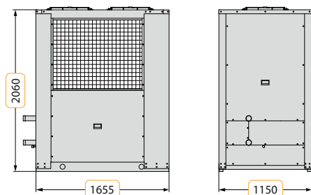
Типоразмеры 045-080
